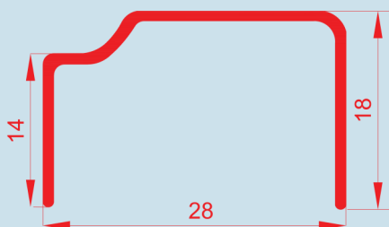
REFUERZO TRASLAPO FIJO R70-003
