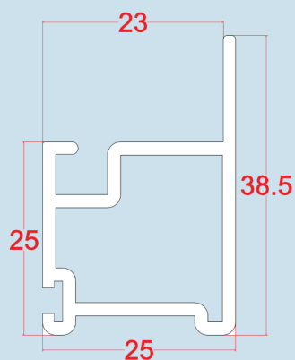
HOJA MOVIL 70-005
