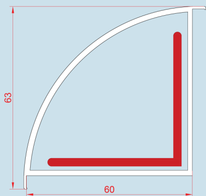
ESQUINERO RODON 90° 70-010
