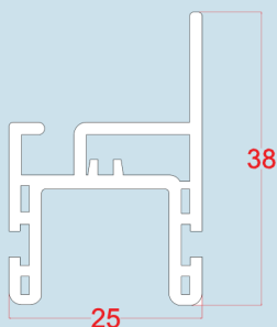
HOJA GUILLOTINA 70-008
