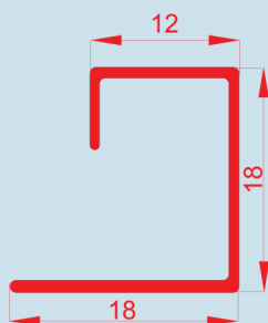
REFUERZO TRASLAPO MOVIL R70-004
