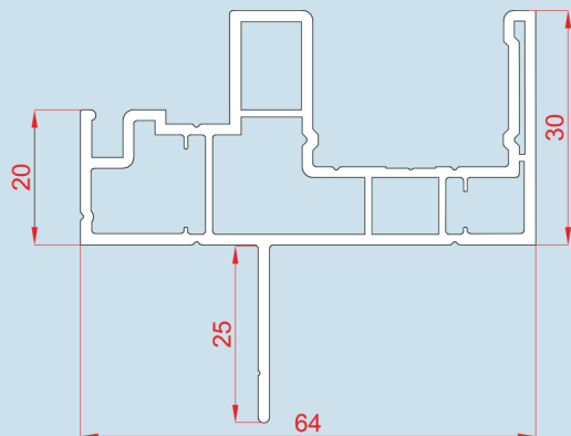
MARCO FIJO 70-001
