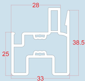
TRASLAPO FIJO 70-003
